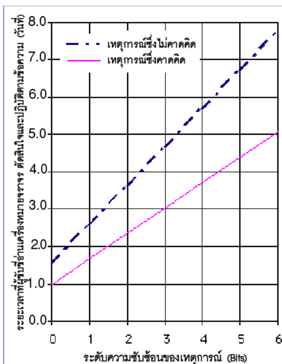
รูปที่ 5-1 แสดงระยะเวลาที่ผู้ขับขี่ใช้ในการอ่านเครื่องหมายจราจร ตัดสินใจและปฏิบัติตามข้อความที่สื่อบนเครื่องหมายจราจรที่ 85 เปอร์เซ็นไทล์
