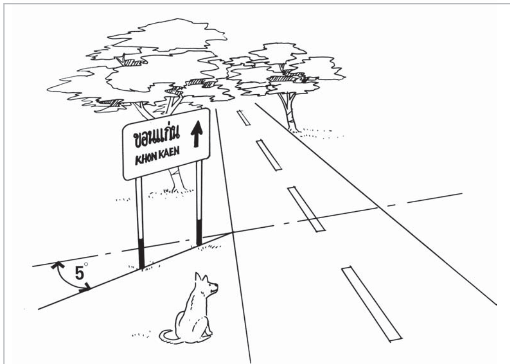
รูปที่ 5-2 ป้ายจราจรควรเบี่ยงจากเส้นตั้งฉากทิศทางจราจรประมาณ 5 องศา
