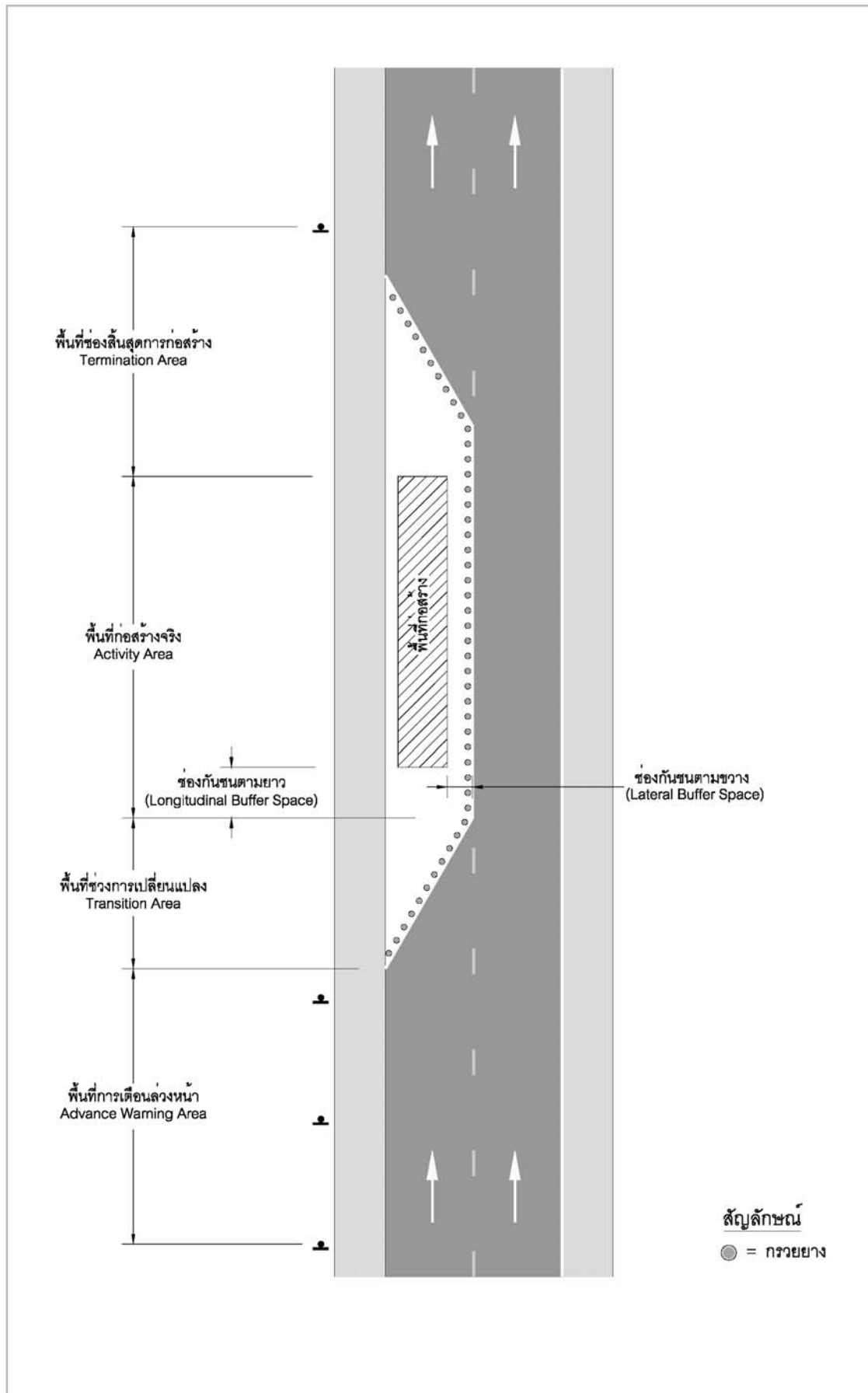
รูปที่ 3-1 การจัดแบ่งพื้นที่บริเวณก่อสร้าง
